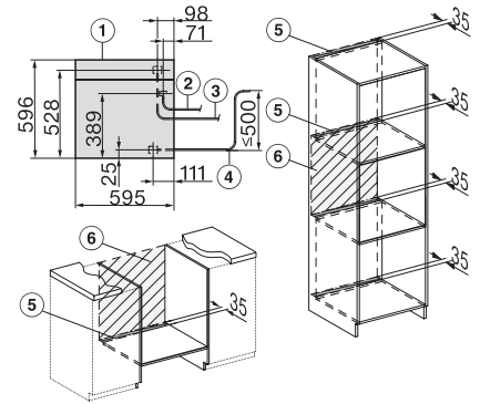
DGC7x65 Anschlüsse und Belüftung 60cm, Skizze
