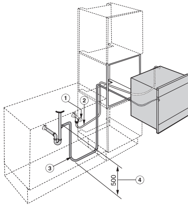
DGC 6000 im Hochschrank, CLST (Skizze)
